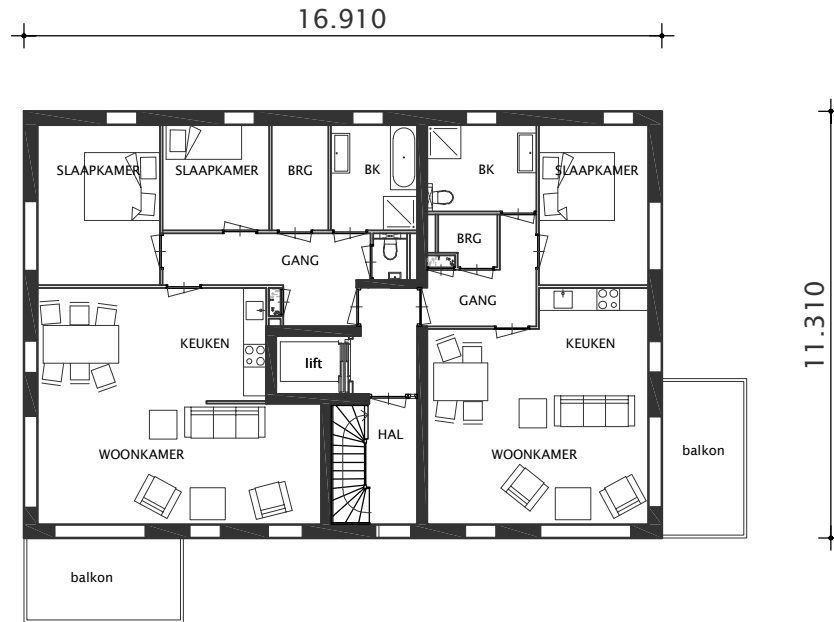
2e verdieping blok B en C
