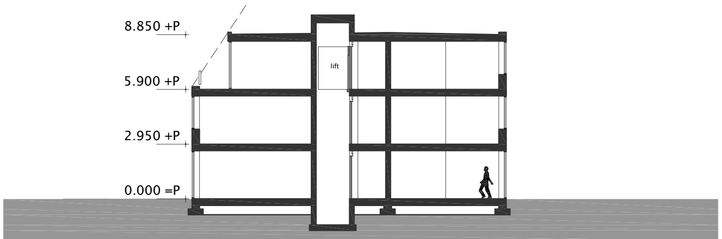
doorsnede blok A (met set-back)
