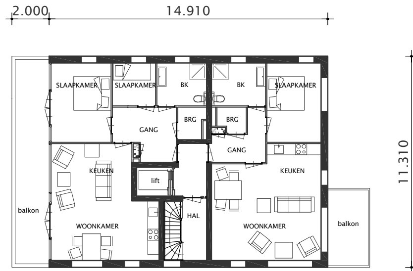
2e verdieping blok A (met set-back)
