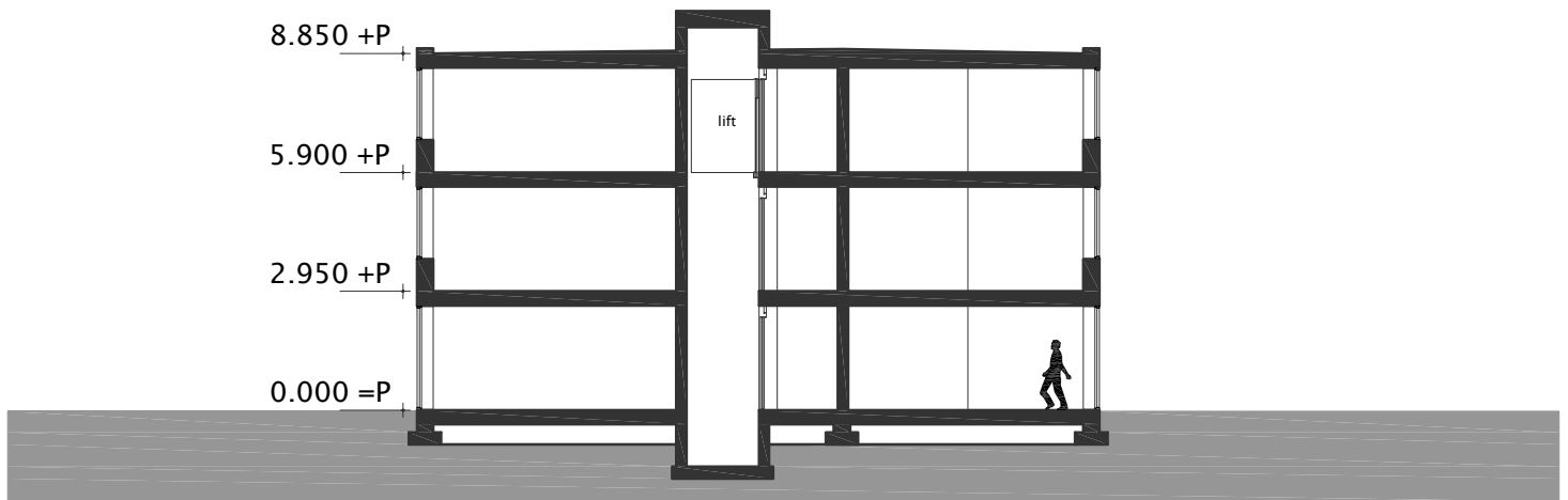
doorsnede blok B en C
